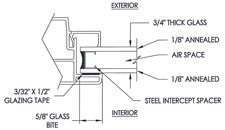
G2 GLAZING DETAIL
