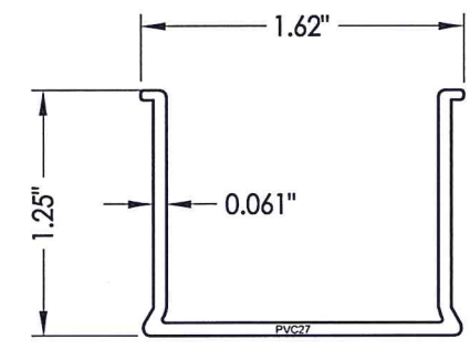
4 FRAME FILLER
