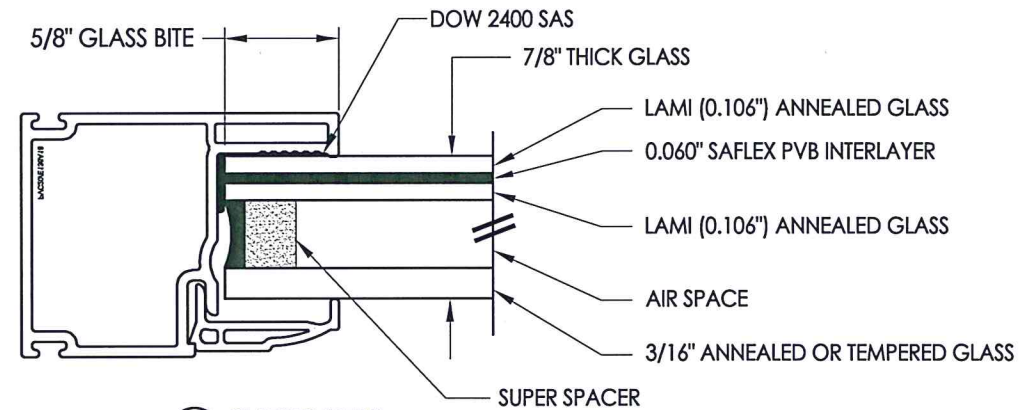
G2 GLAZING DETAIL
