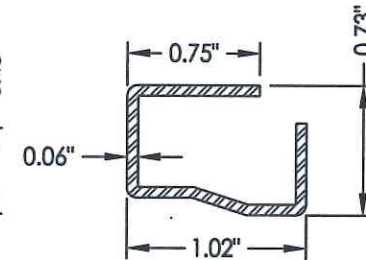
17 REINFORCEMENT MED Stiles
