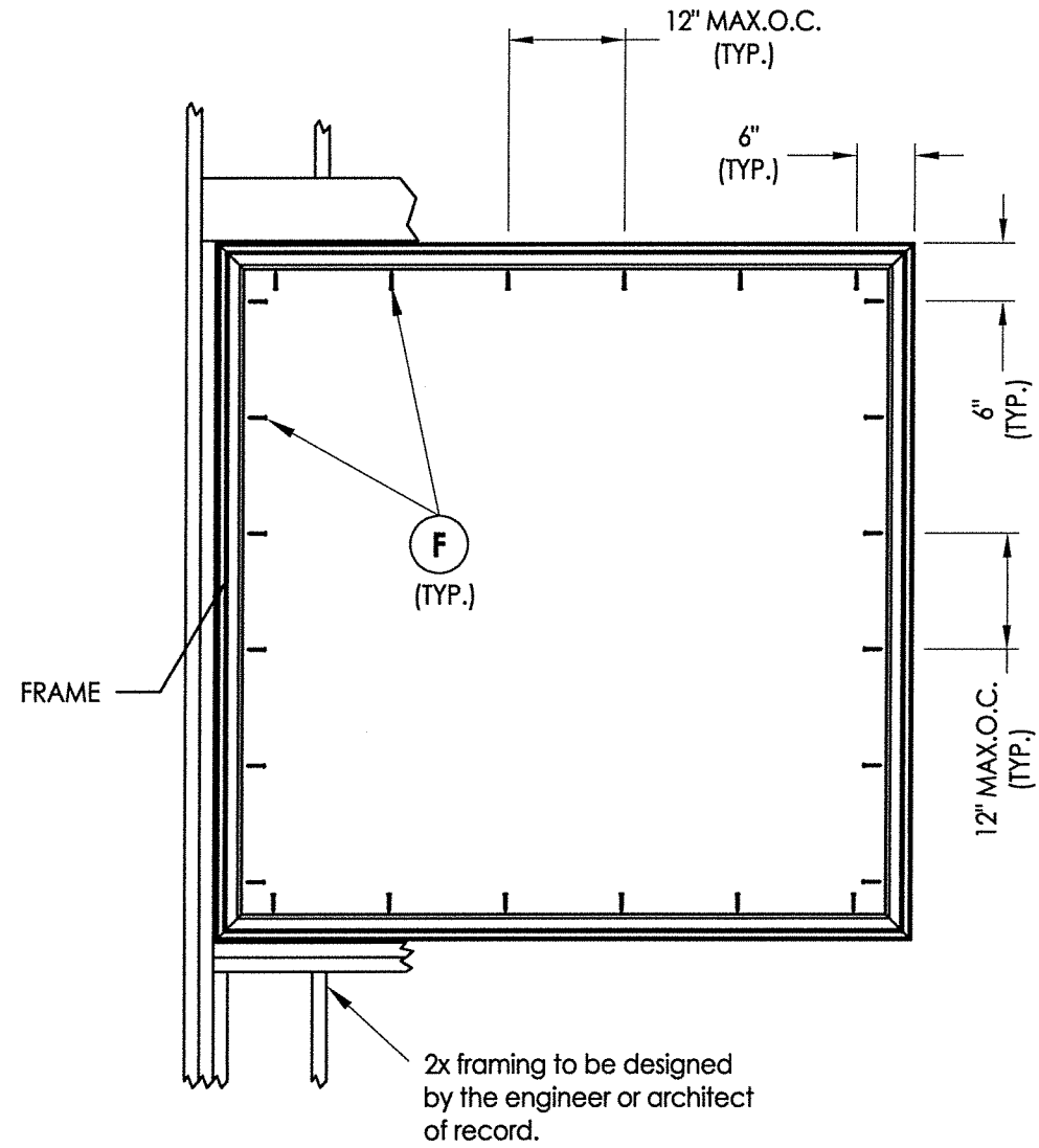
FRAME ANCHORING 72" X 72" MAX
