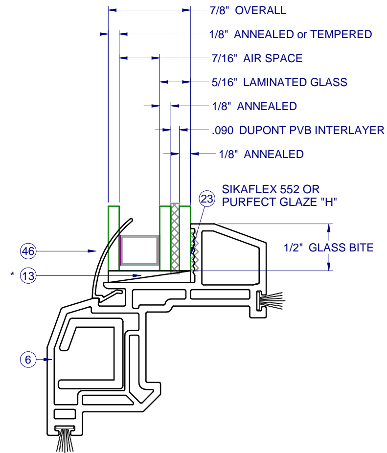
ELEVATION B
