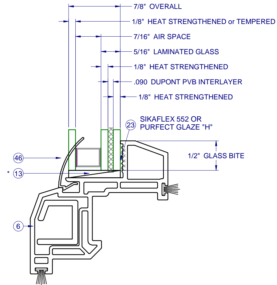
ELEVATION A
