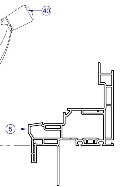
ALTERNATE FIN FRAME
