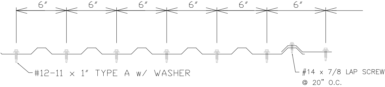
6"-6"-6"-6"-6"-6" SCREW PATTERN
