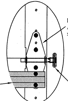
TYPICAL END HINGE N.T.S. ③
