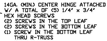
TYPICAL CENTER HINGE N.T.S. 2
