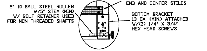
TYPICAL BOTTOM BRACKET N.T.S. 4
