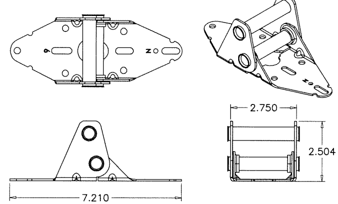
#6 HINGE (11 GA. STEEL)
