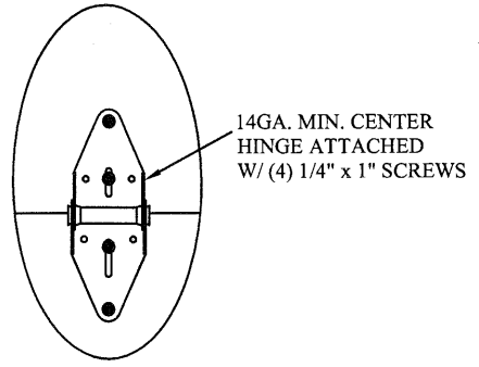
TYPICAL CENTER HINGE N.T.S. 2
