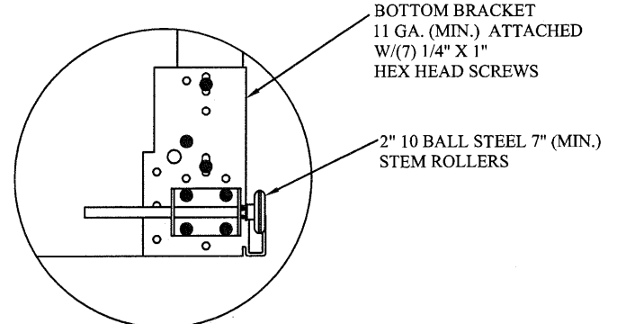
TYPICAL BOTTOM BRACKET N.T.S. 4
