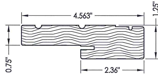
1 POLY FIBER JAMB
