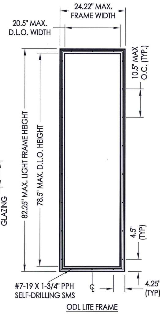
3A ODL LITE FRAME Aluminum
