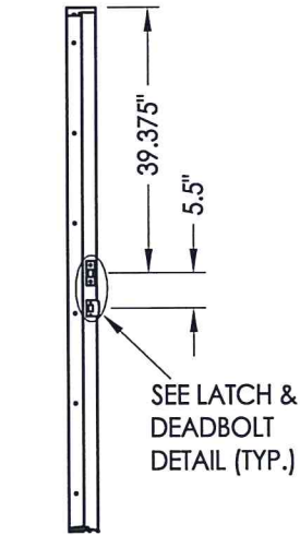
STRIKE JAMB
