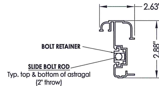
63 ASTRAGAL DLP
