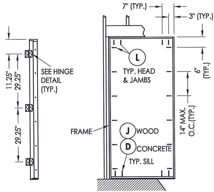
HINGE JAMB
