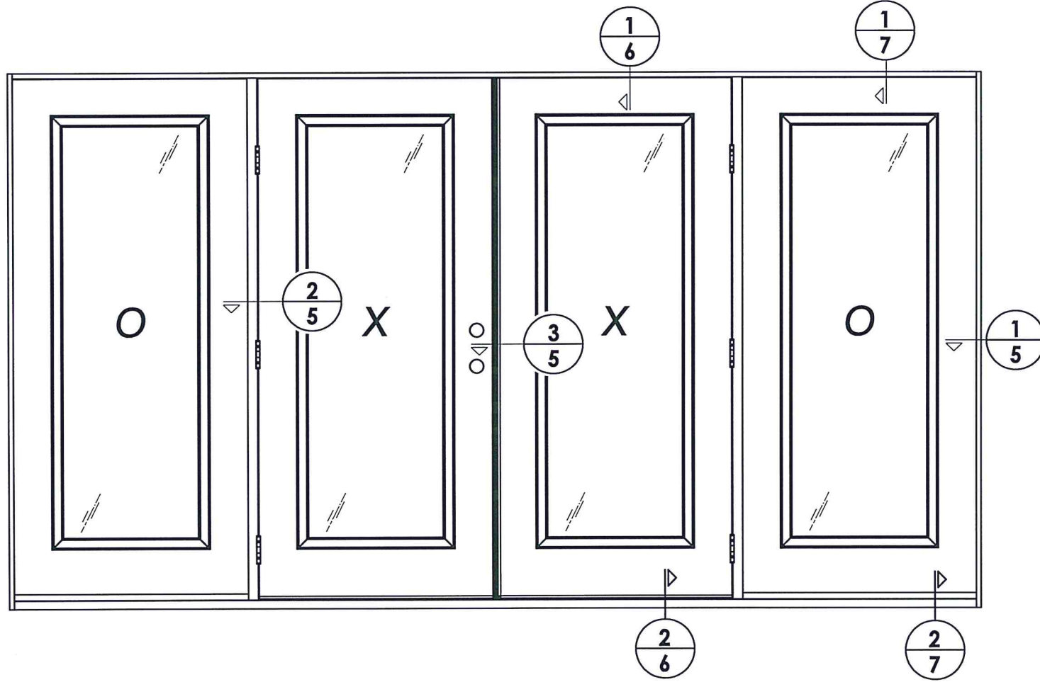
ELEVATION (OXXO)
