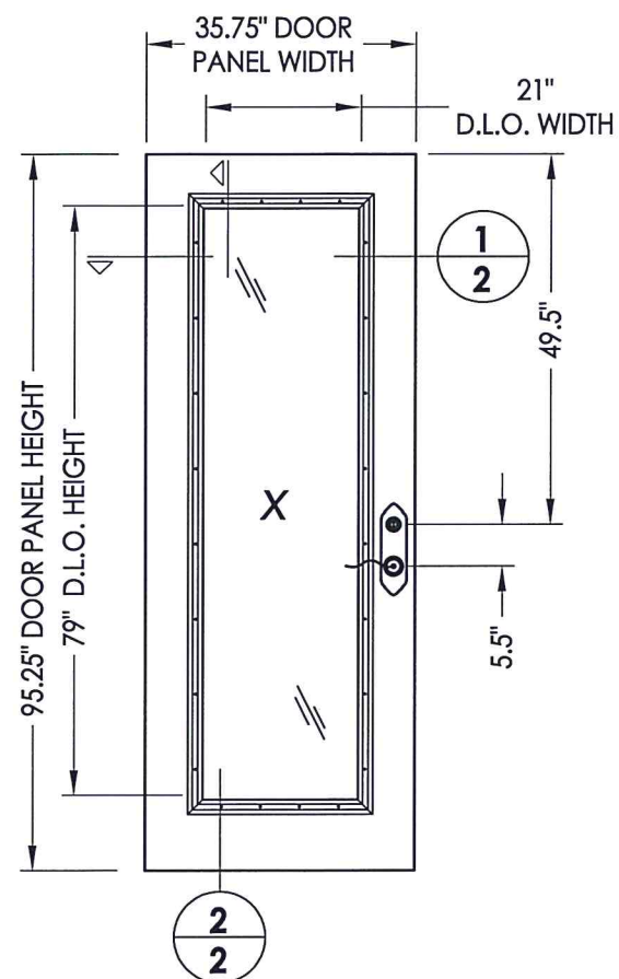
40 DOOR PANEL
