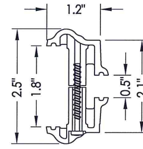
3F PLASTIC LIP LITE FRAME ODL
