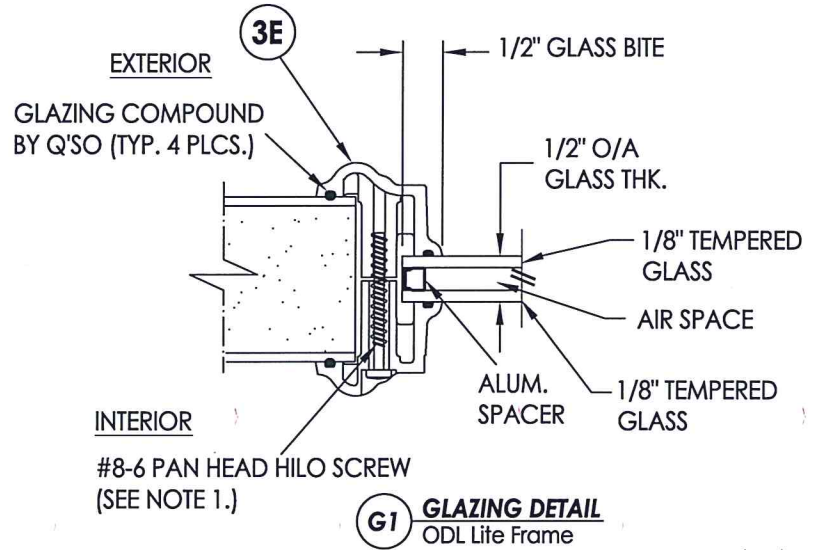
3E PLASTIC LIP LITE FRAME ODL
