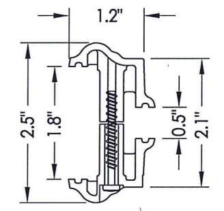
3E PLASTIC LIP LITE FRAME ODL
