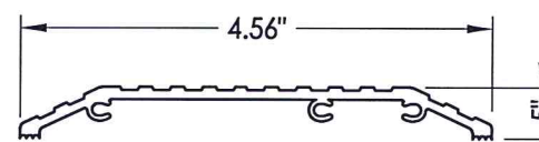
71 ADA SILL
