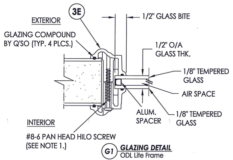
3E PLASTIC LIP LITE FRAME ODL
