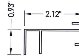
29 SIDELITE SPACER
