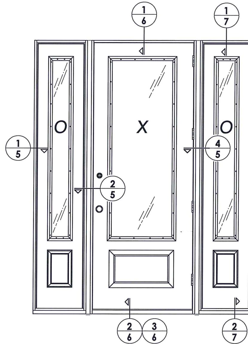
ELEVATION (OXO)
