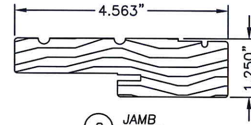
9 8 JAMB
