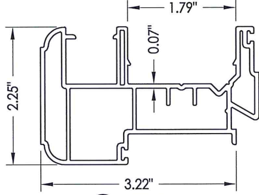
38 ASTRAGAL Exterior
