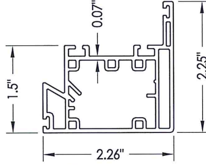
37 ASTRAGAL Exterior
