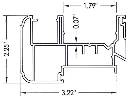
38 ASTRAGAL Exterior
