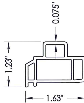
9 RISER
