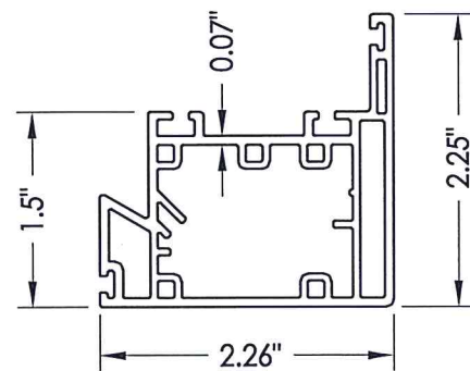
37 ASTRAGAL Exterior
