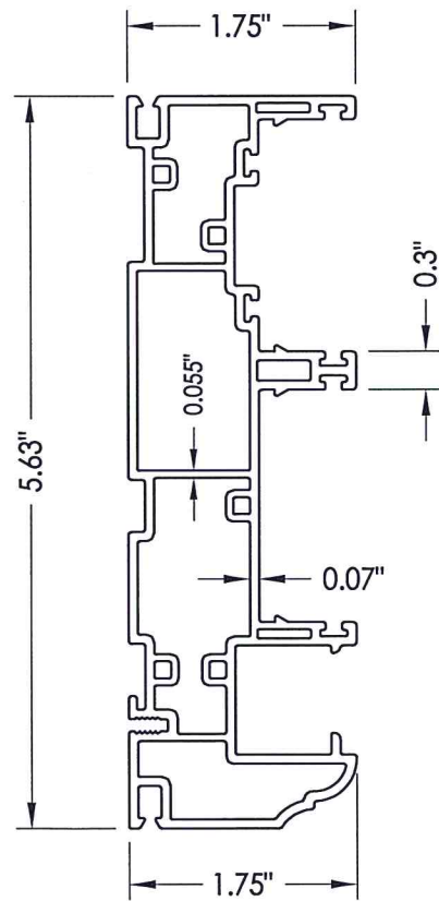
6 PD JAMB
