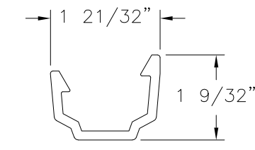
T-ASTRAGAL RIGID PVC
