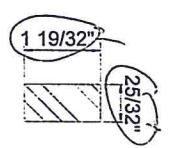
10 REIN. WOOD-(D) Wood
