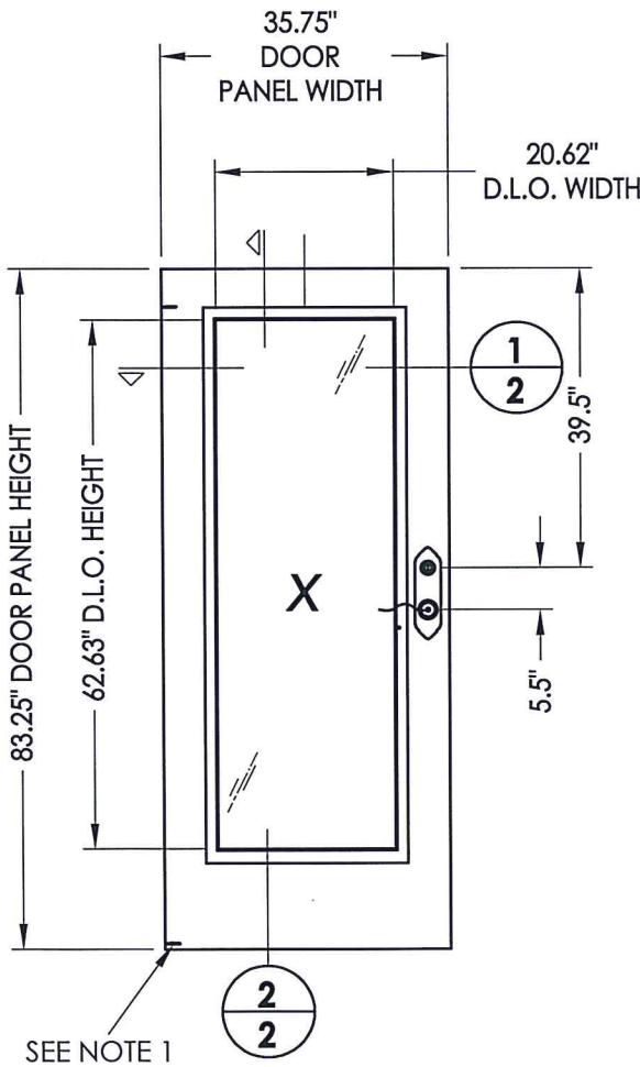
40 DOOR PANEL
