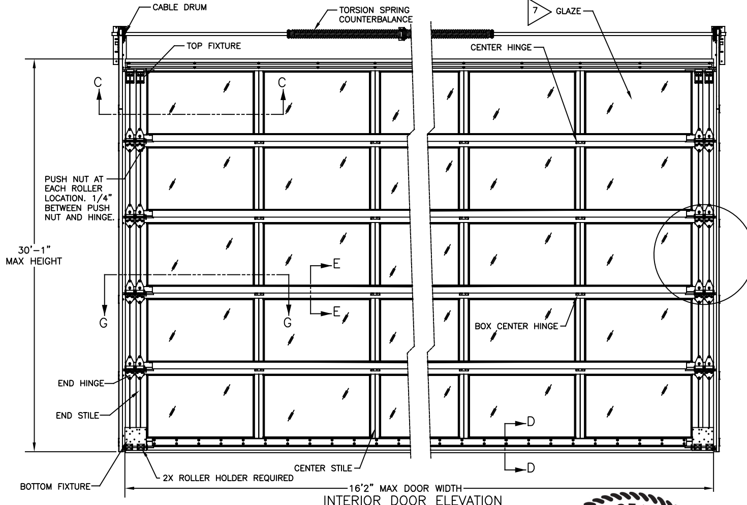
16'2" MAX DOOR WIDTH 30'-1" MAX HEIGHT INTERIOR DOOR ELEVATION
