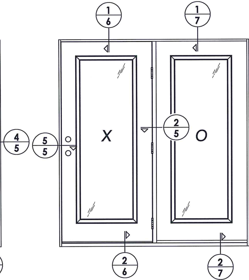
ELEVATION (XO - OX) center hinge
