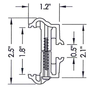
3F PLASTIC LIP LITE FRAME ODL
