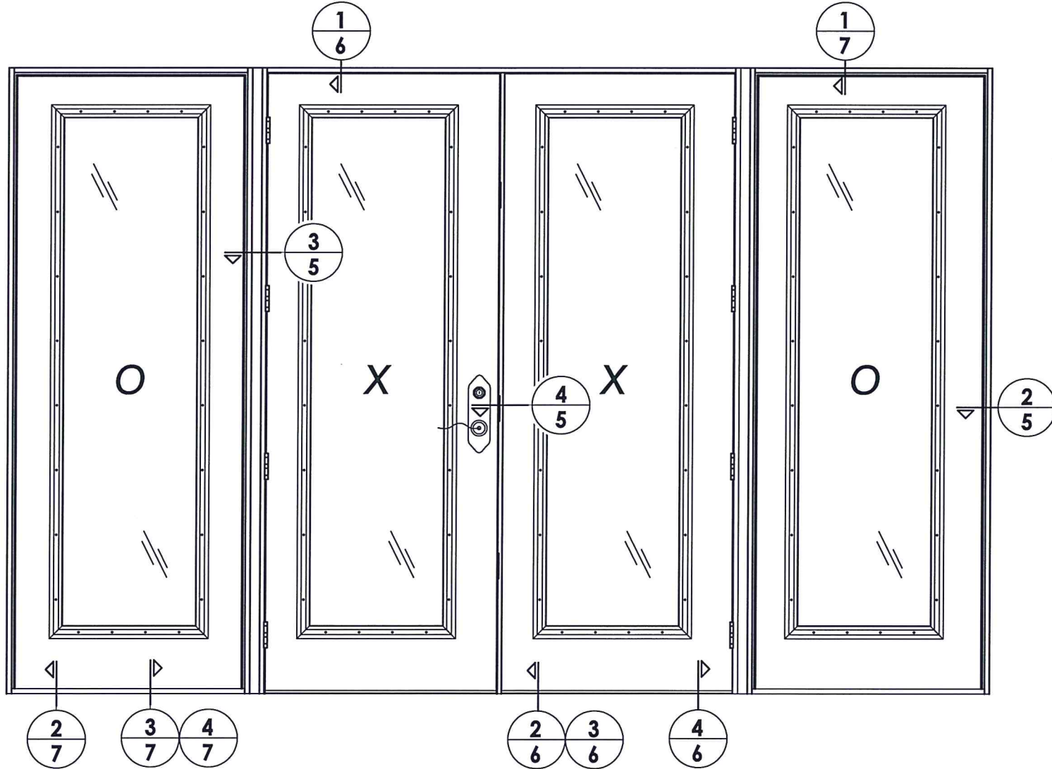
ELEVATION (OXXO)
