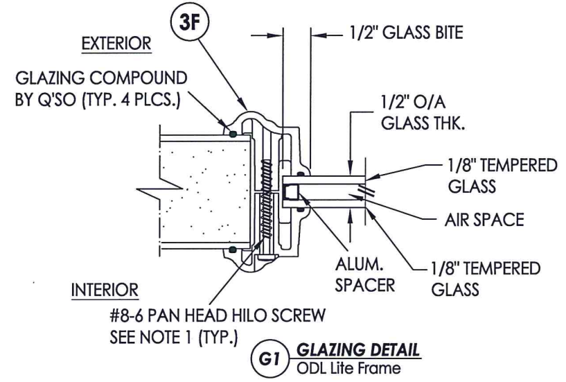
3F PLASTIC LIP LITE FRAME ODL
