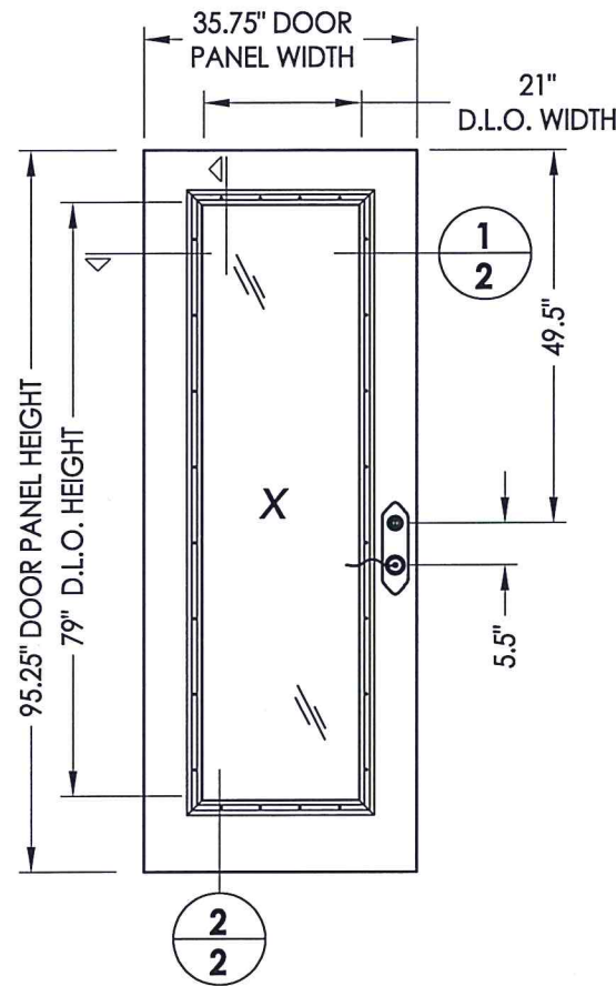
40 DOOR PANEL
