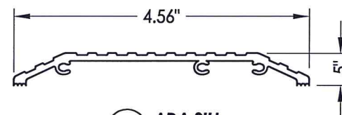
71 ADA SILL
