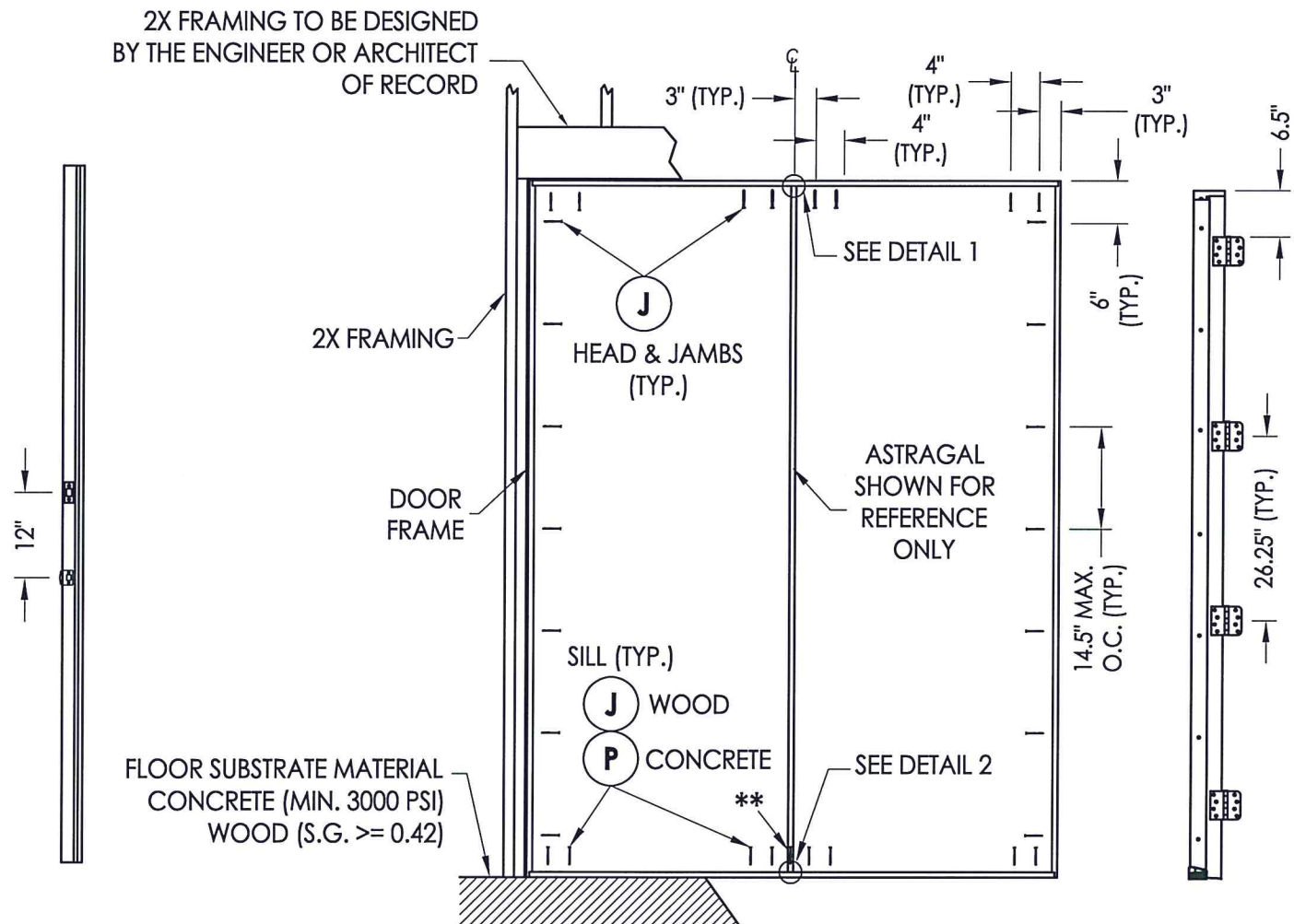
ASTRAGAL
