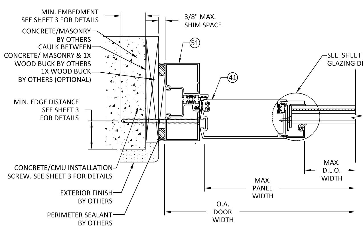
A HORIZONTAL SECTION 6 500T DOOR & TRIFAB 451T SUBFRAME JAMB-CONCRETE/CMU
