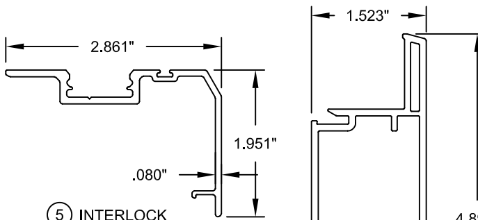
5 INTERLOCK
