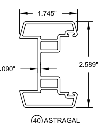
40 ASTRAGAL
