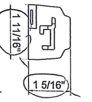
25 ASTRAGAL BOTTOM CAP RIGID PVC
